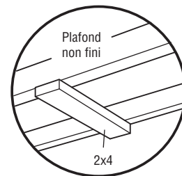
MONTAGE DU SUPPORT DE LINTEAU AU PLANFOND EN OPTION
